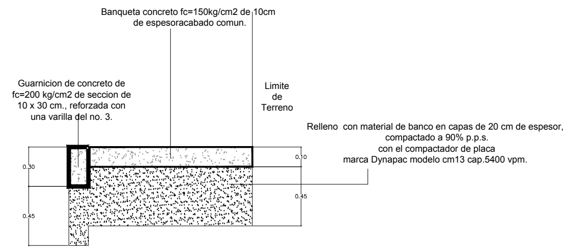
DETALLE CONSTRUCTIVO DE BANQUETA
