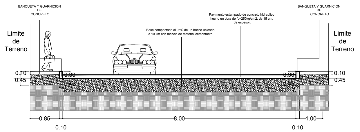
DETALLE CONSTRUCTIVO DE CALLE.
