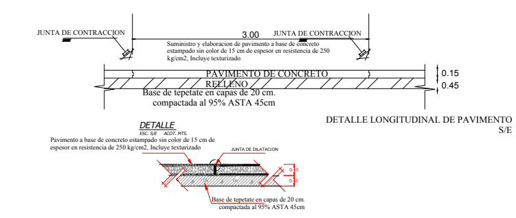
DETALLE CONSTRUCTIVO DE BANQUETA
